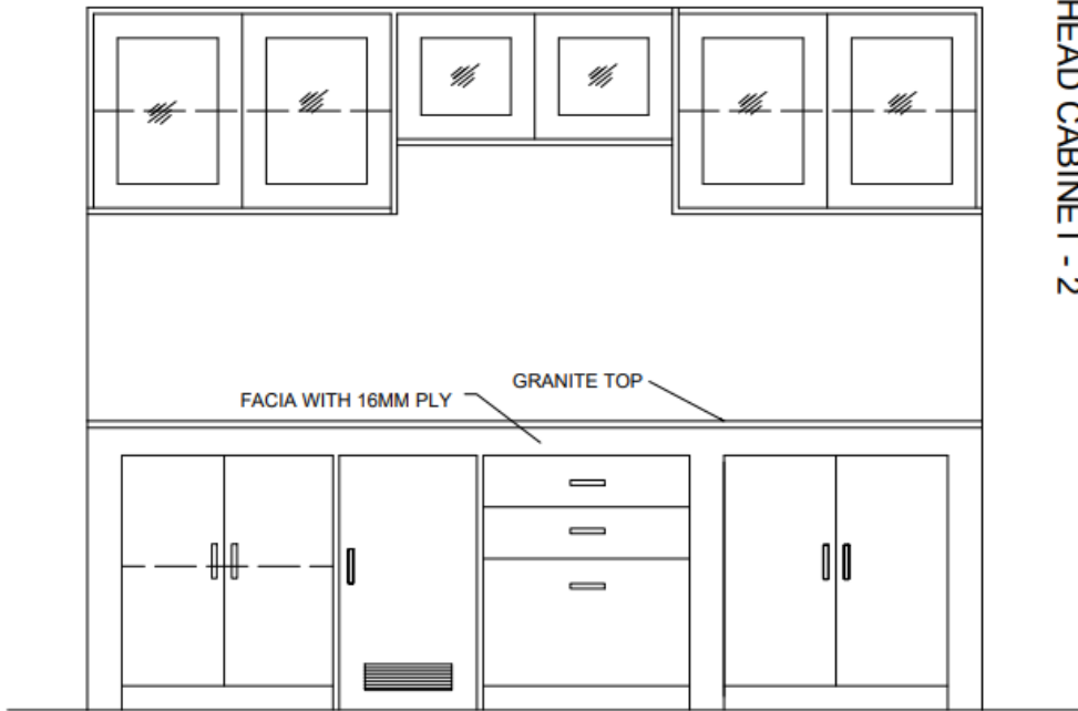
ELEVATION
